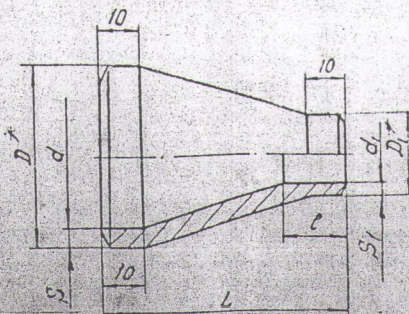
*Размеры для справок Рисунок 10
